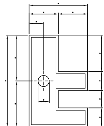
Rinne in L-Form mit 1 Stichkanal
